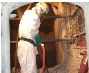
焼却炉解体作業(レベル2)
