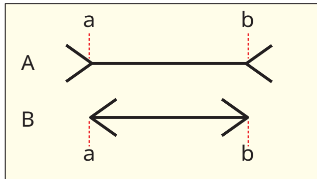
図2 錯視の例
